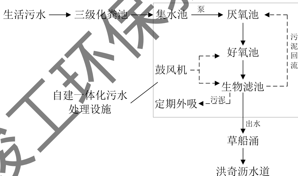
图3-1 项目污水处理工艺流程图
